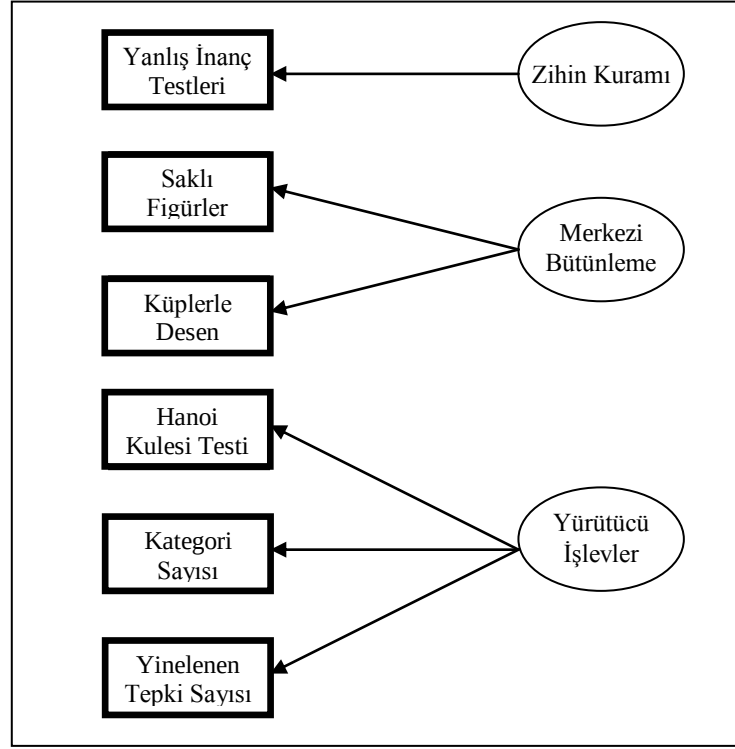
Şekil 3. Ölçme modeli
